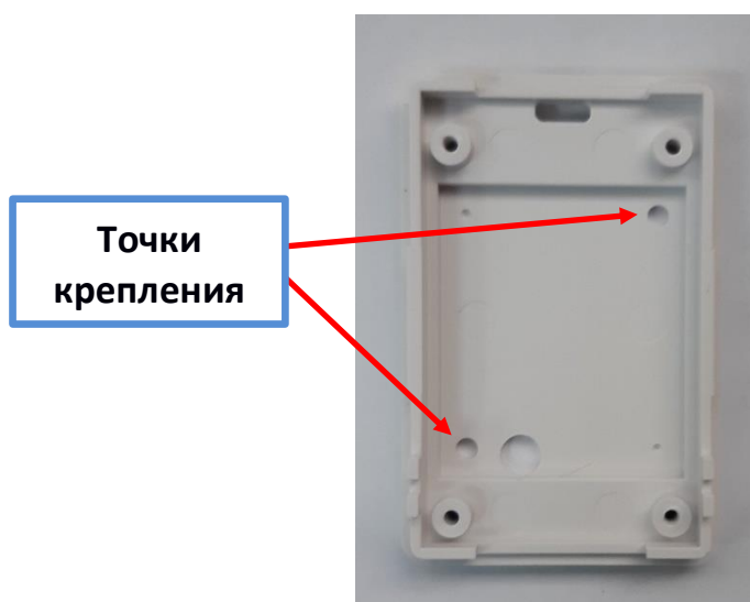
Рис. 17 – Точки крепления модулей
