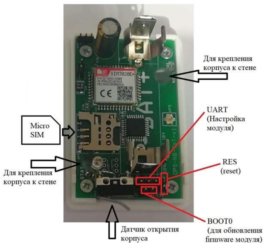
Рис. 2 – Расположение технологического разъема XP1 и джамперов RES,BOOT0.
